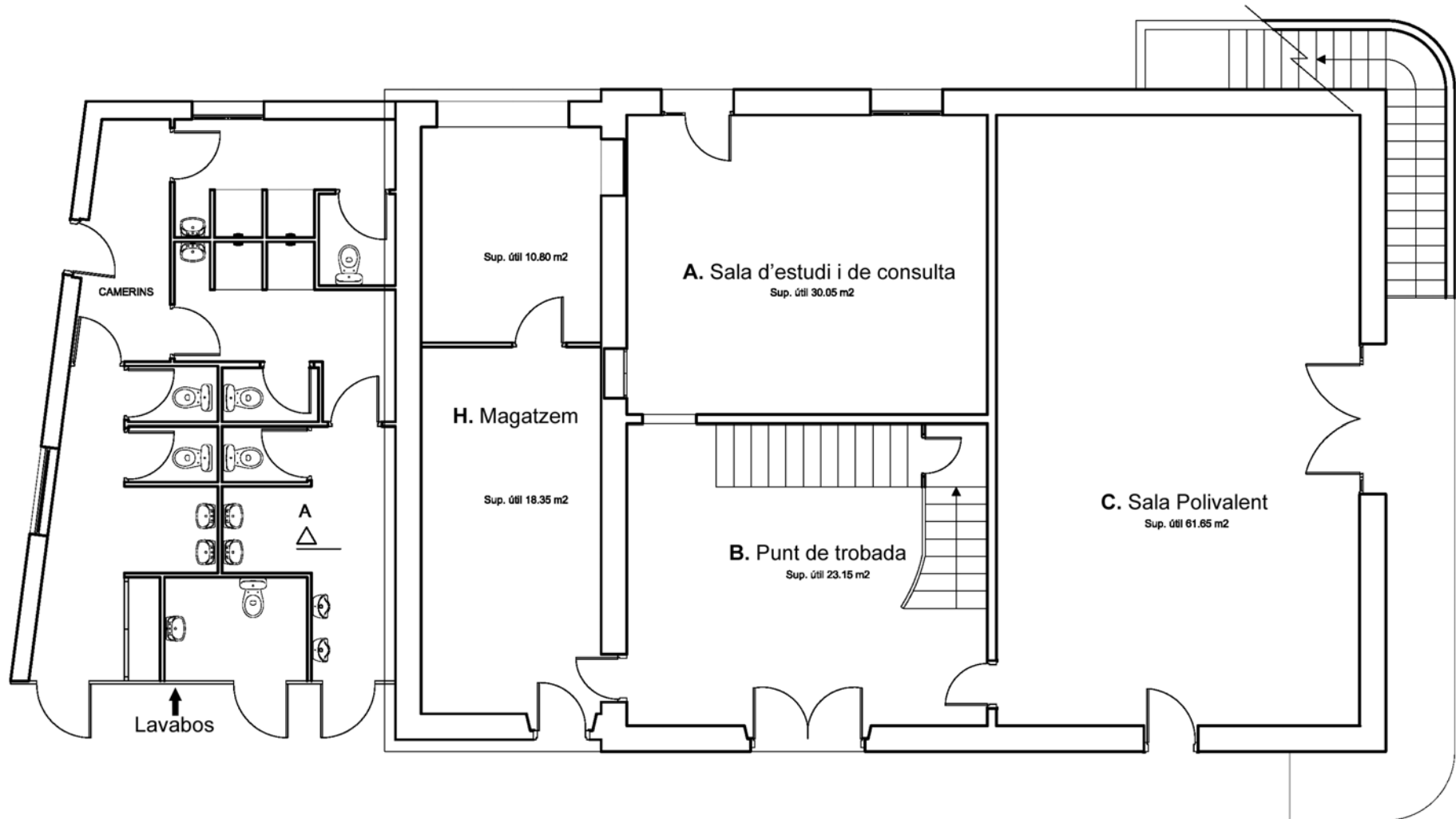
Plànol 1. Planta baixa i usos
