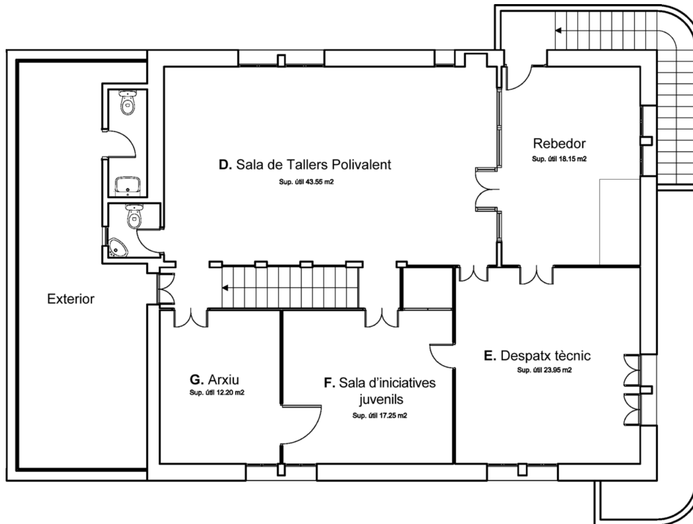
Plànol 2. Primera planta i usos
